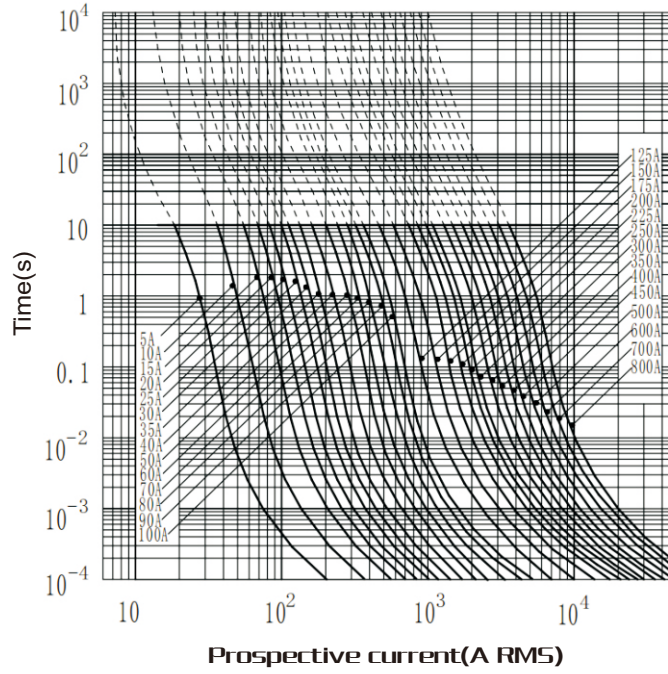
Current Characteristics 时间电流特性图
