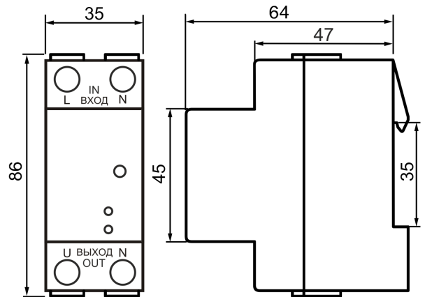
Габаритные размеры
