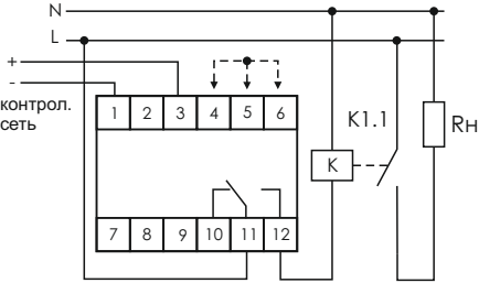
R н - защищаемая установка К - контактор
