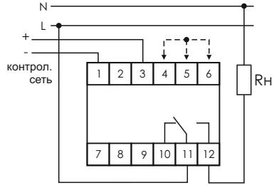
R н - защищаемая установка
